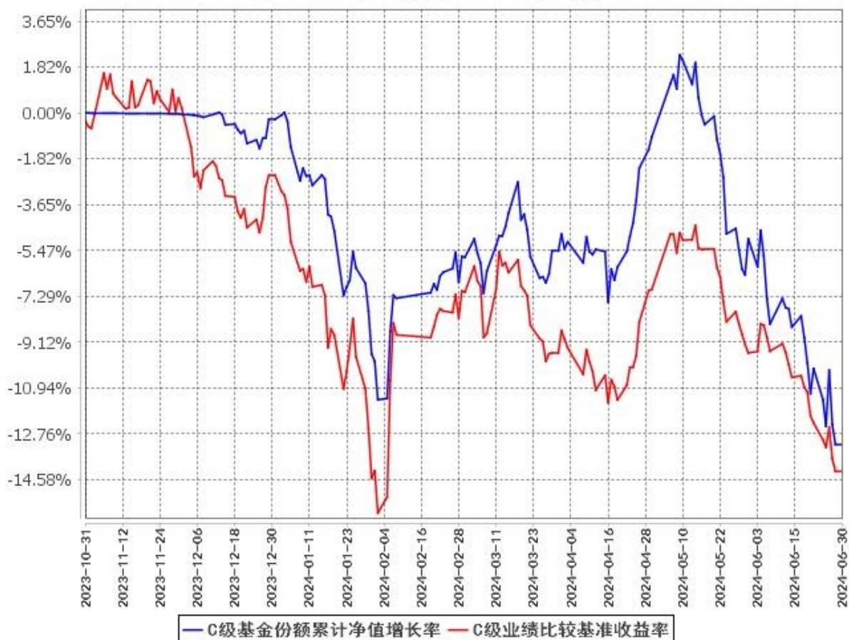
C级基金份额累计净值增长率与同期业绩比较基准收益率的历史走势对比图 (2023年10月31日至2024年6月30日)
