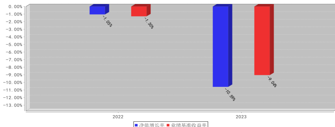
东方红多元策略混合C基金每年净值增长率与同期业绩比较基准收益率的对比图（2023年12月31日）
