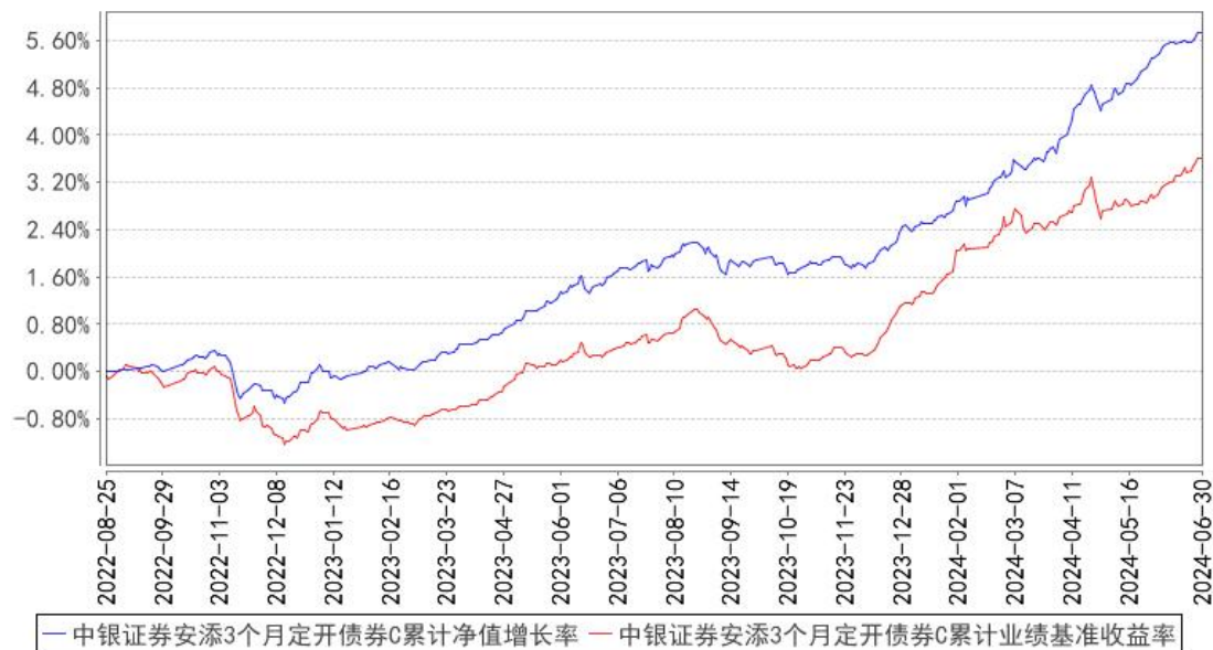
中银证券安添3个月定期开债券C累计净值增长率与同期业绩比较基准收益率的历史走势对比图
