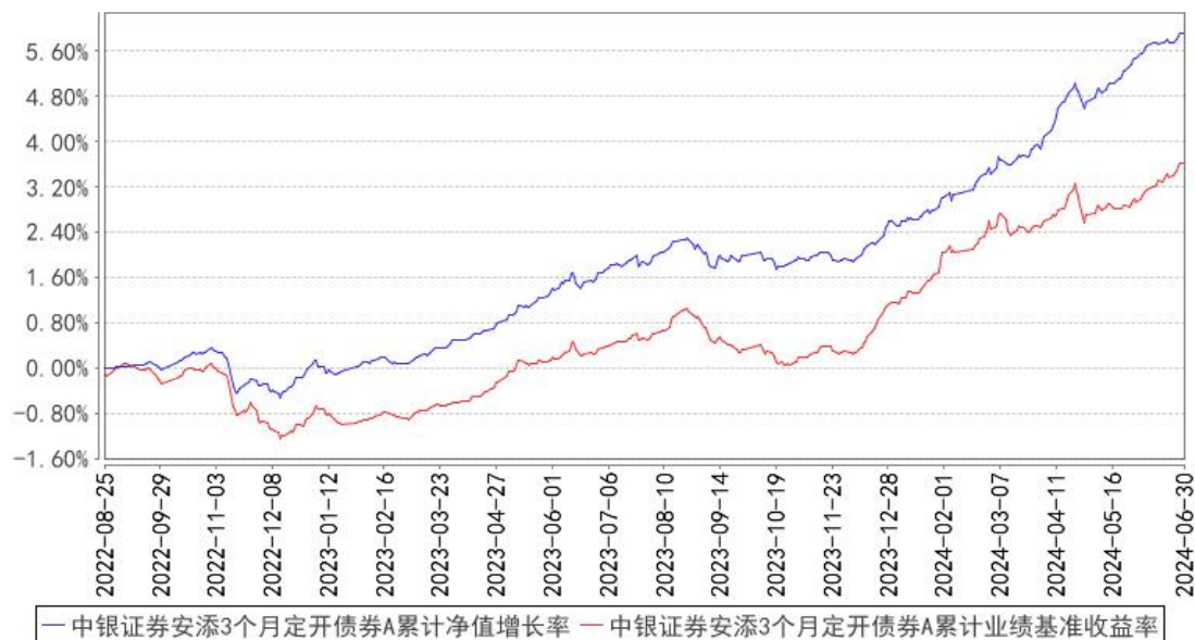
中银证券安添3个月定期开债券A累计净值增长率与同期业绩比较基准收益率的历史走势对比图
