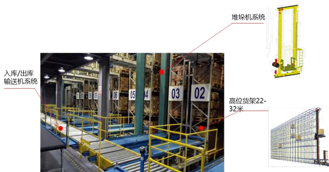
图 14-17 自动仓储系统存取系统构成示意图
