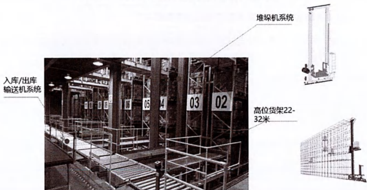
图 2-17 自动仓储系统存取系统构成示意图
