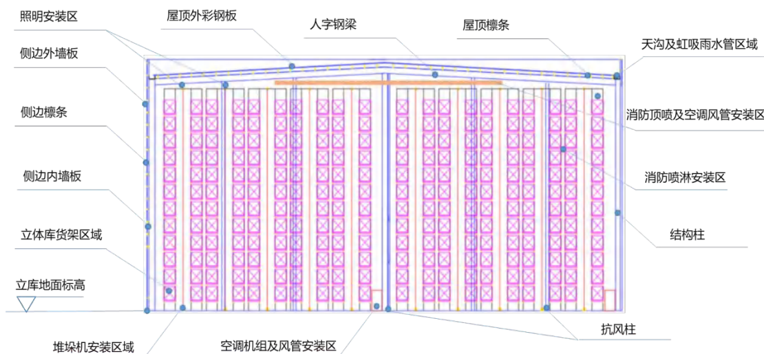
图2-14 立体库内部结构
