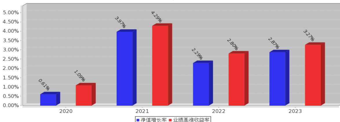
嘉实彭博国开债 1-5 年指数 C 基金每年净值增长率与同期业绩比较基准收益率的对比图（2023 年 12 月 31 日）
