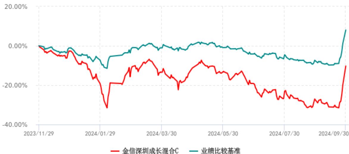
金信深圳成长混合C累计净值增长率与业绩比较基准收益率历史走势对比图 (2023年11月29日-2024年09月30日)
