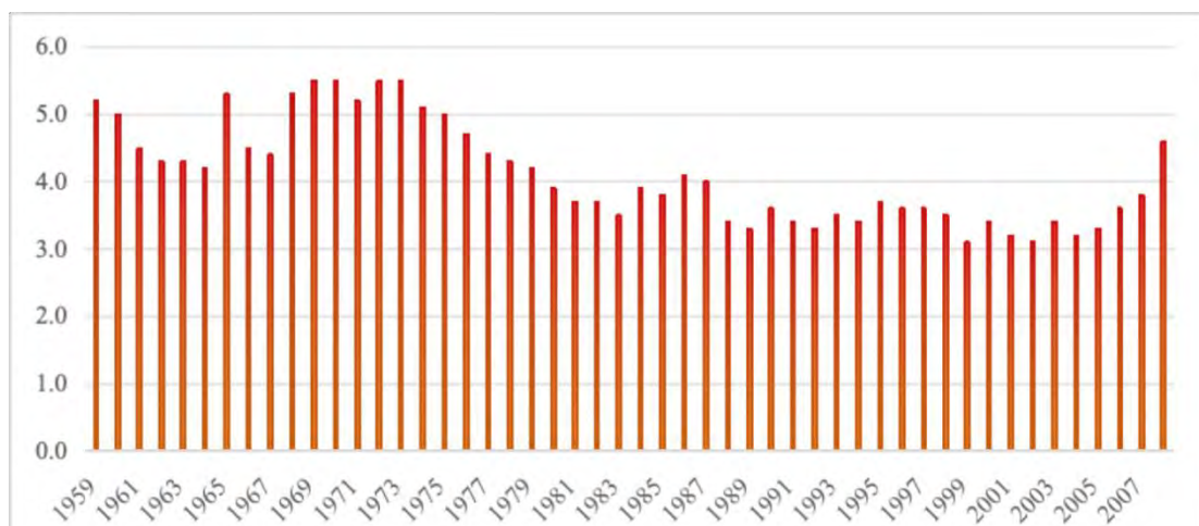
图 14-12 察右中旗气象站 1959—2008 年 10m 高度平均风速年际变化图
