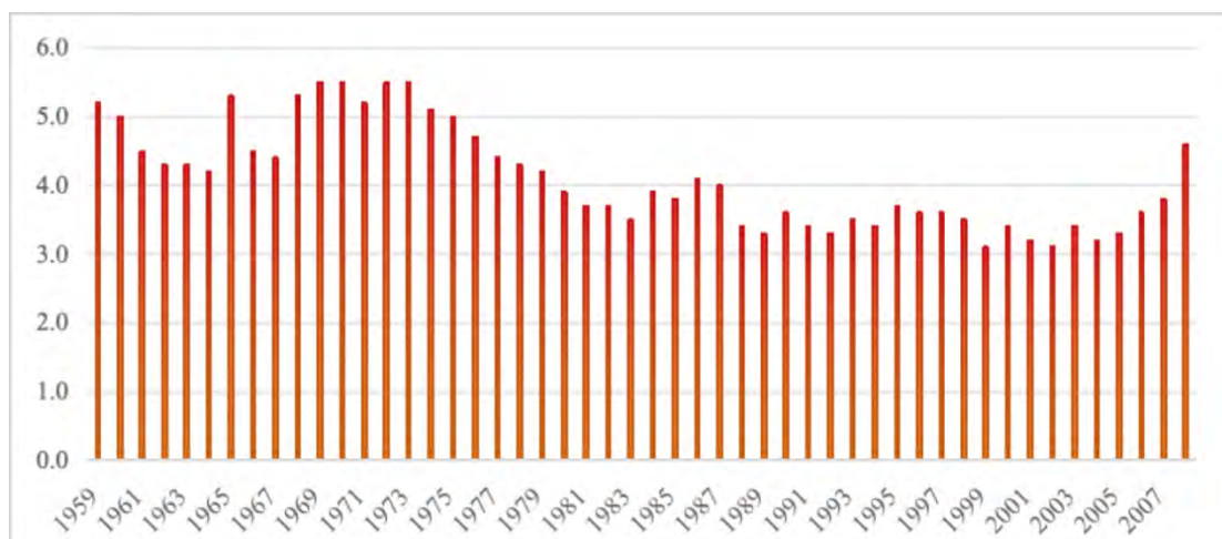
图 3-12 察右中旗气象站 1959—2008 年 10m 高度平均风速年际变化图(m/s)
