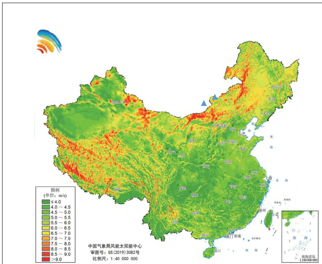
图 3-6 2023 年全国陆地 70 米高度年平均风速分布图
