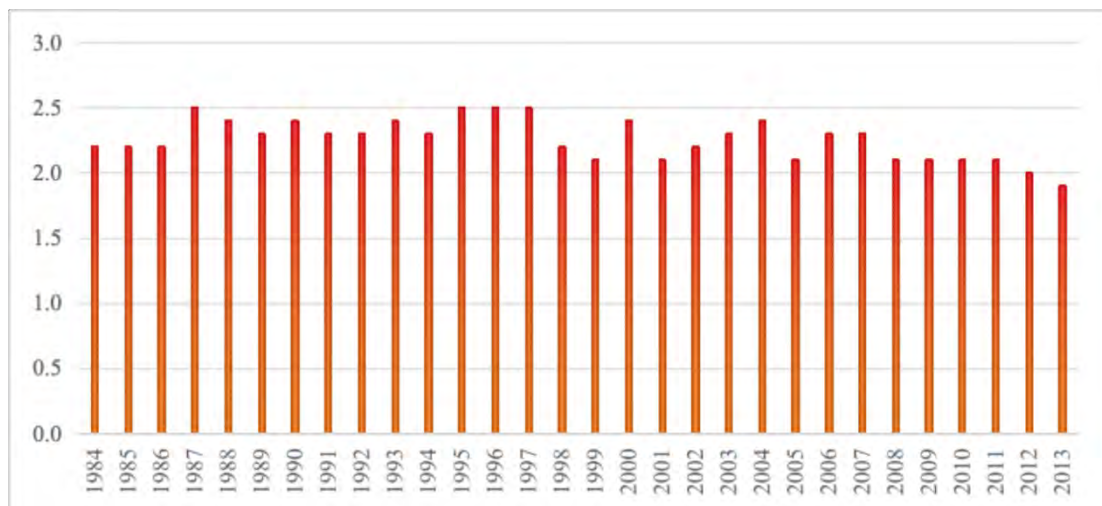
图 3-11 固阳县气象站 1984—2013 年 10m 高度平均风速年际变化图（m/s）
