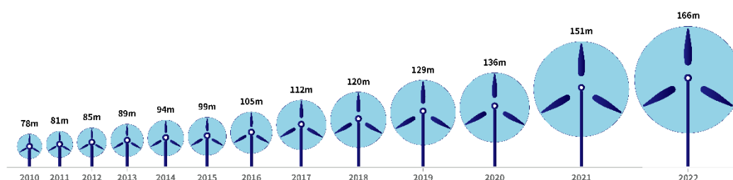
2008-2022 年国内新增陆上风电装机叶轮直径变化趋势
