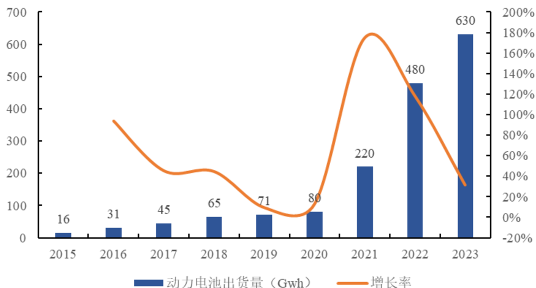
2015-2023年我国动力电池出货量及增长率
