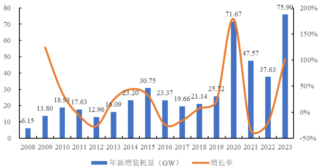
2008-2023我国风机年新增装机量
