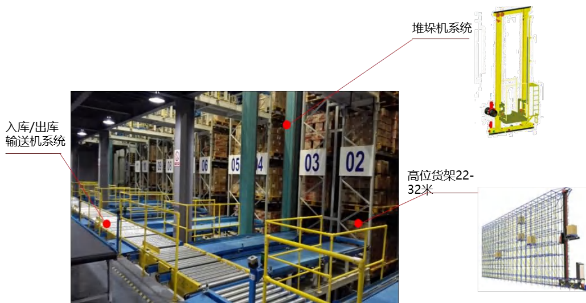
图2-16 自动仓储系统存取系统构成示意图
