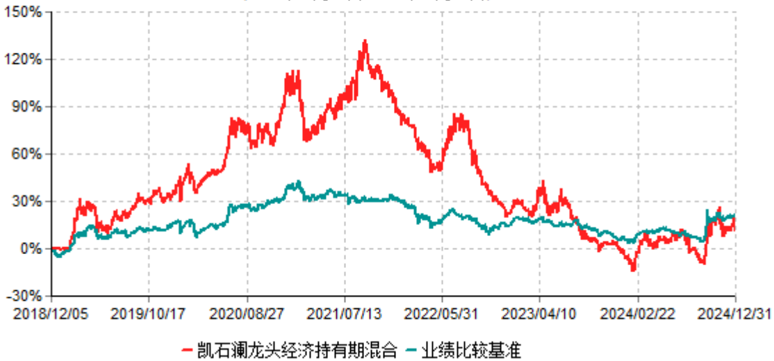
凯石澜龙头经济一年持有期混合型证券投资基金累计净值增长率与业绩比较基准收益率历史走势对比图 (2018年12月05日-2024年12月31日)
