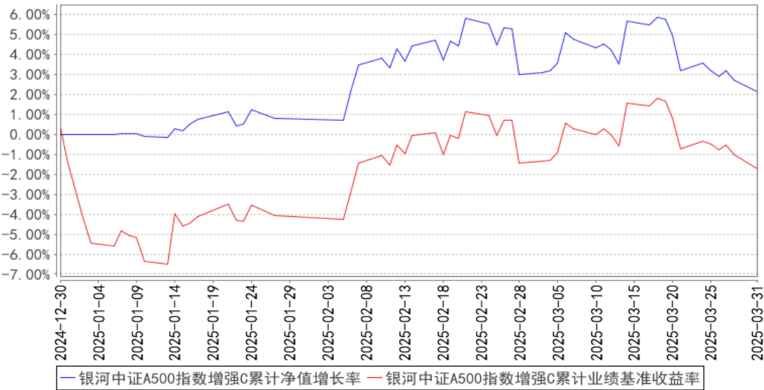
银河中证A500指数增强C累计净值增长率与同期业绩比较基准收益率的历史走势对比图
