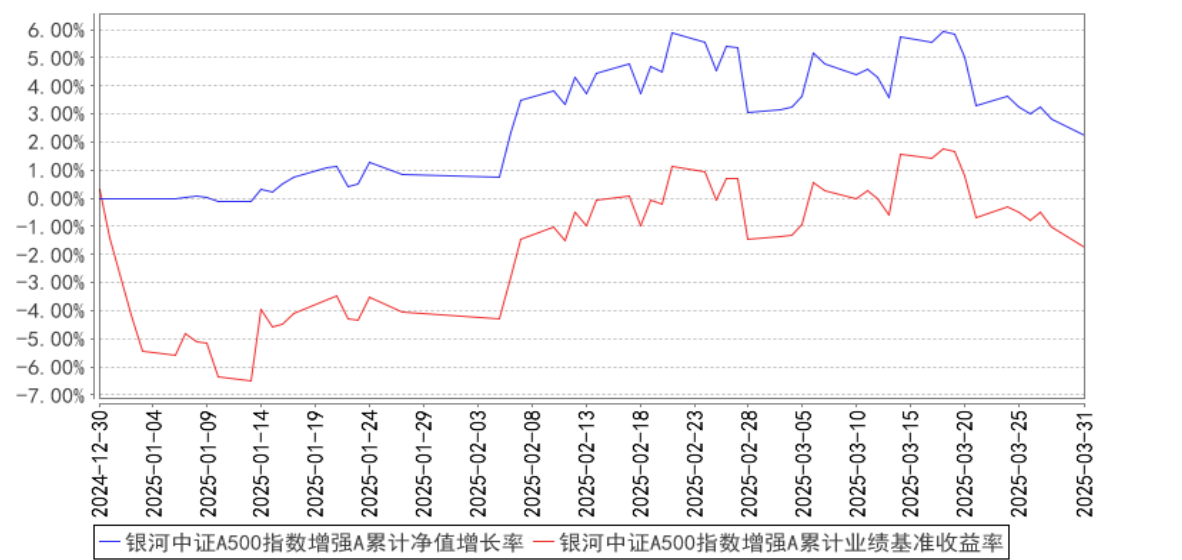
银河中证A500指数增强A累计净值增长率与同期业绩比较基准收益率的历史走势对比图
