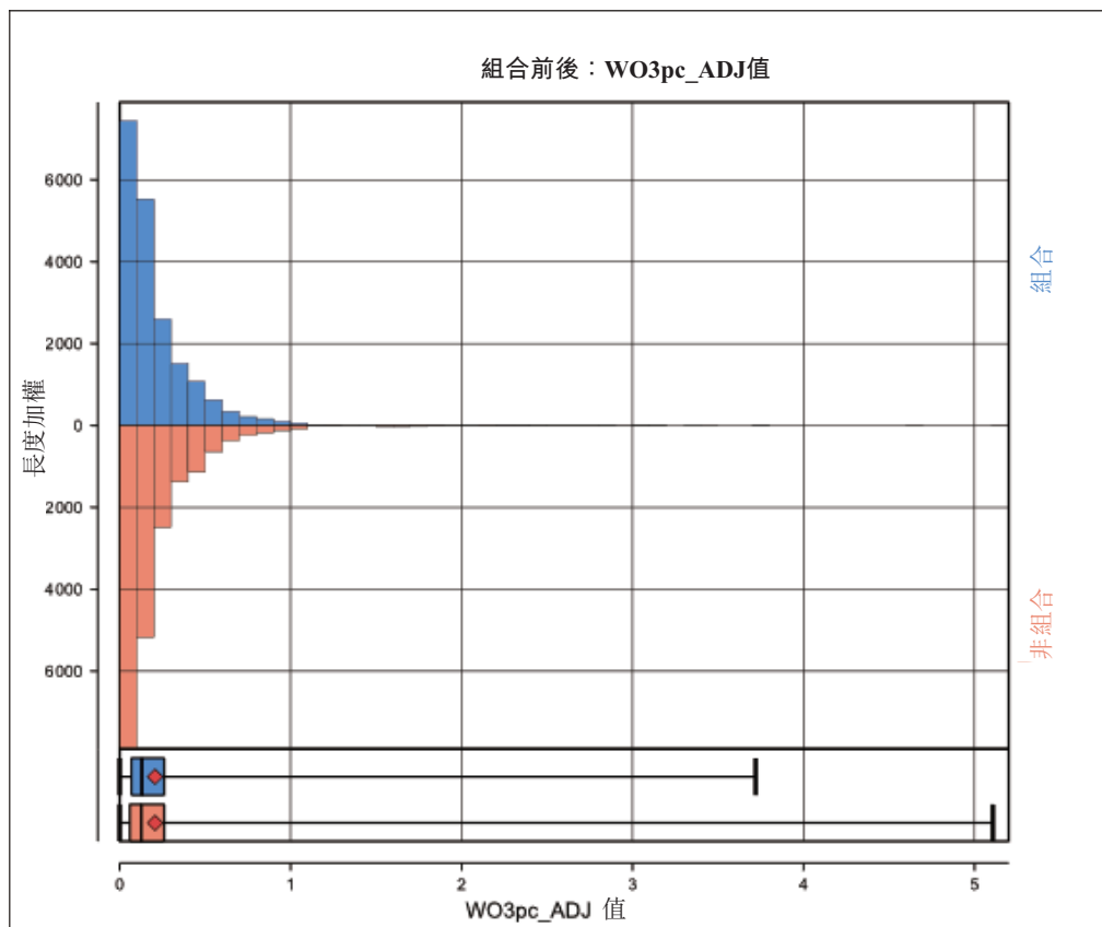
圖5.4：組合和原始樣品的頻率統計數據－資源區域
