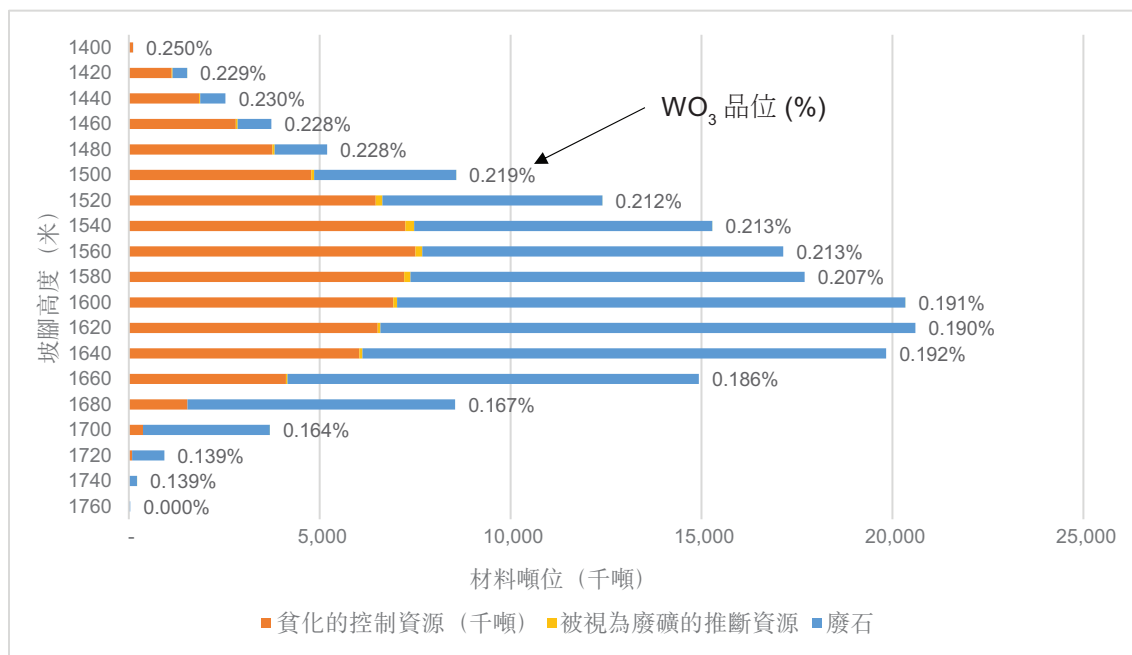
圖6.8：露天礦設計中的逐台材料
