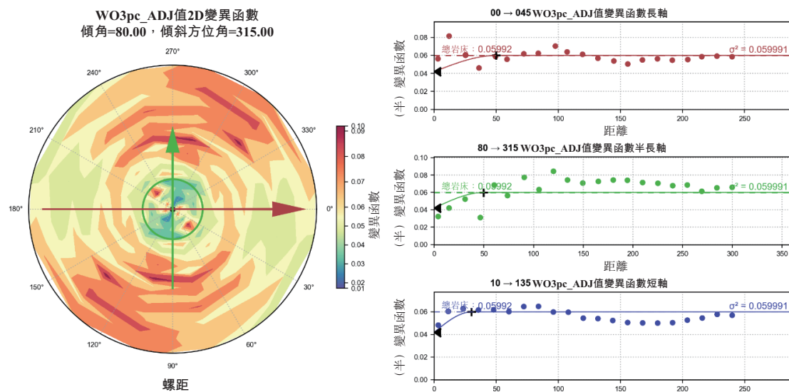
圖5.6：變異函數圖和適配模型－資源區域
