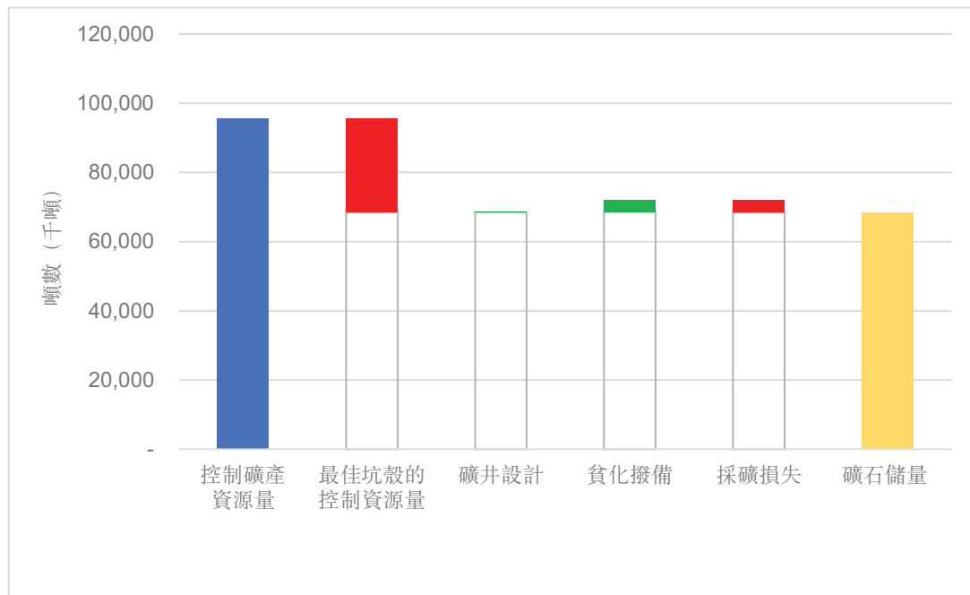
圖6.13：採礦存貨的瀑布圖
