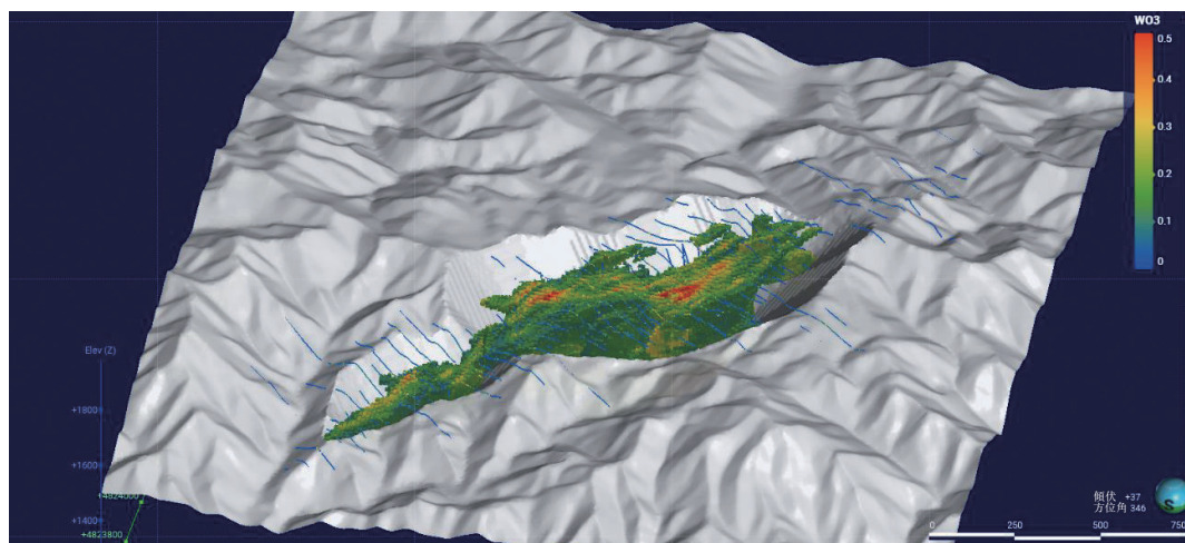
圖5.14：概念坑殼內的礦產資源分佈
