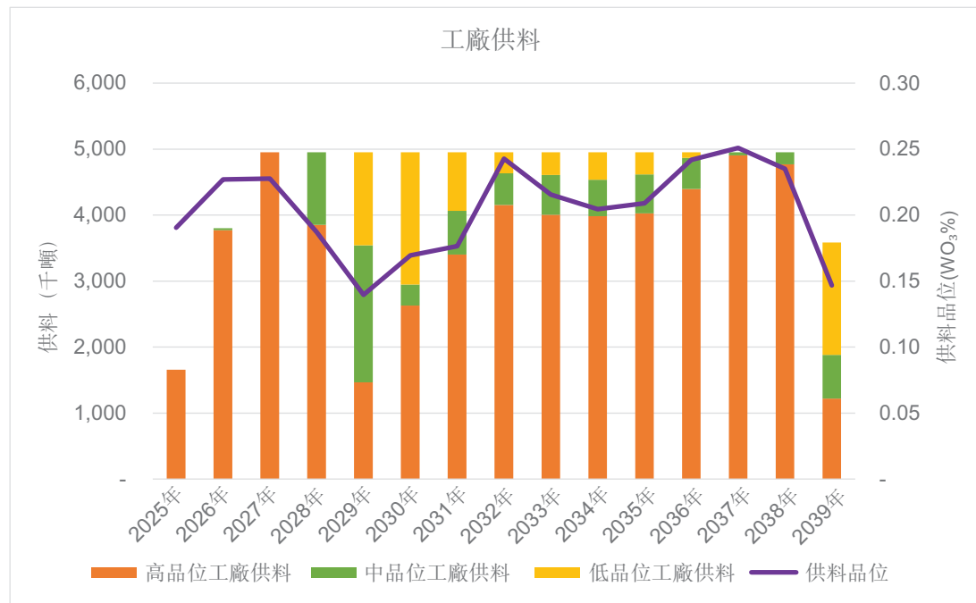
圖6.11：礦山服務年限的工廠供料時間表
