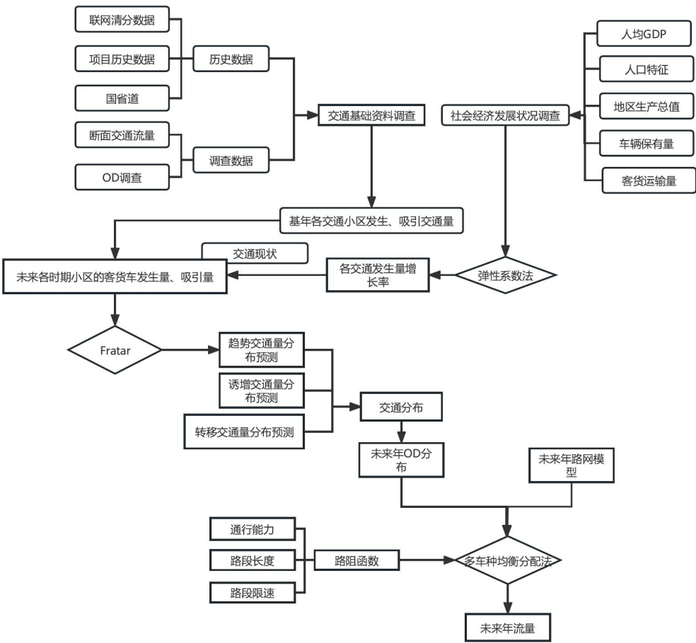
图 16-1 预测流程图
