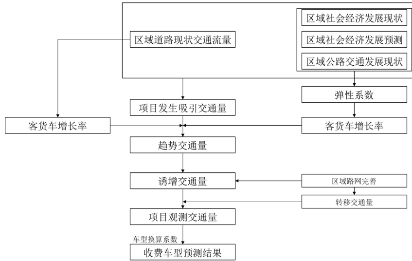
图 16-1 预测流程图
