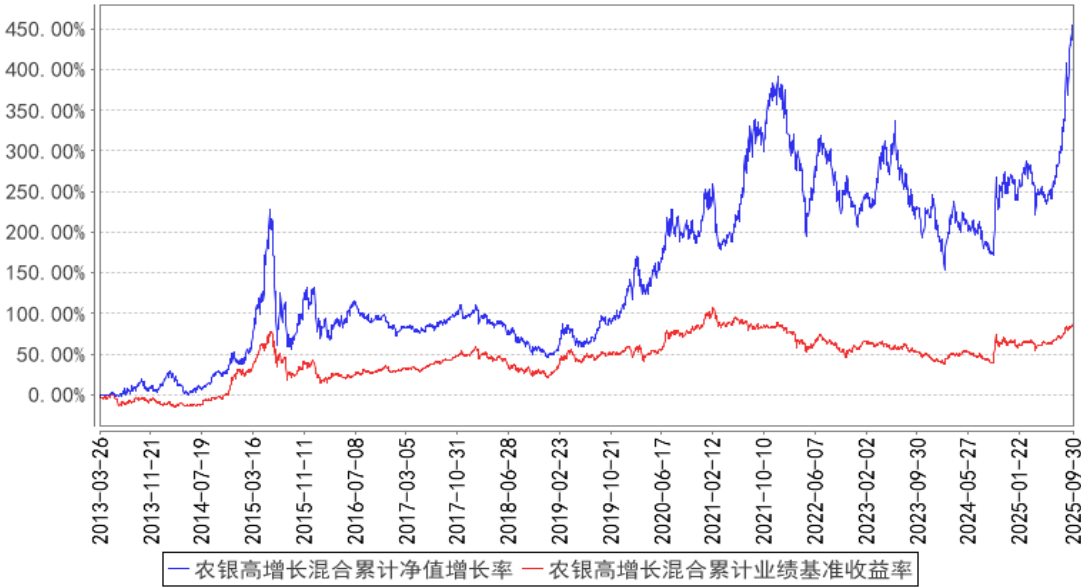
农银高增长混合累计净值增长率与同期业绩比较基准收益率的历史走势对比图
