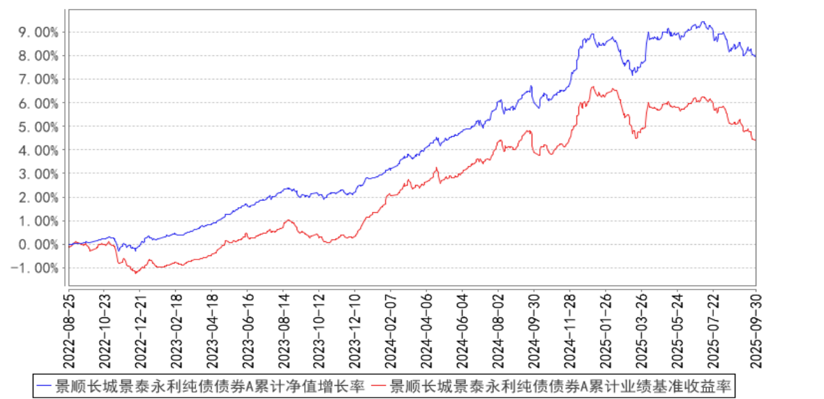
景顺长城景泰永利纯债债券A累计净值增长率与同期业绩比较基准收益率的历史走势对比图
