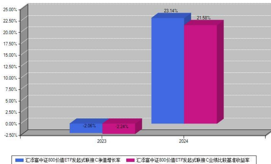
汇添富中证800价值ETF发起式联接C每年净值增长率与同期业绩基准收益率对比图
