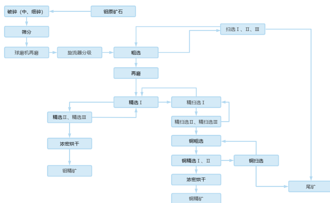
选矿流程
