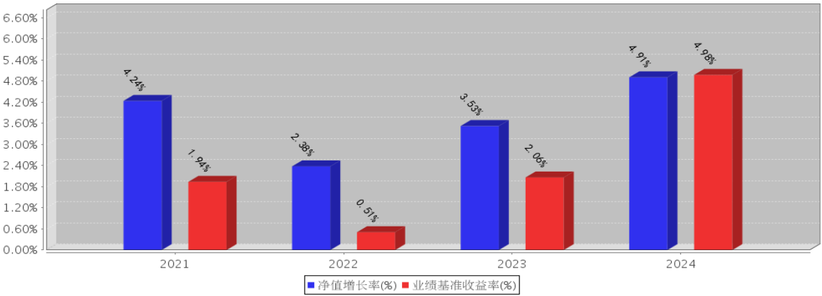
景顺长城景泰恒利一年定开债券基金每年净值增长率与同期业绩比较基准收益率的对比图（2024年12月31日）
