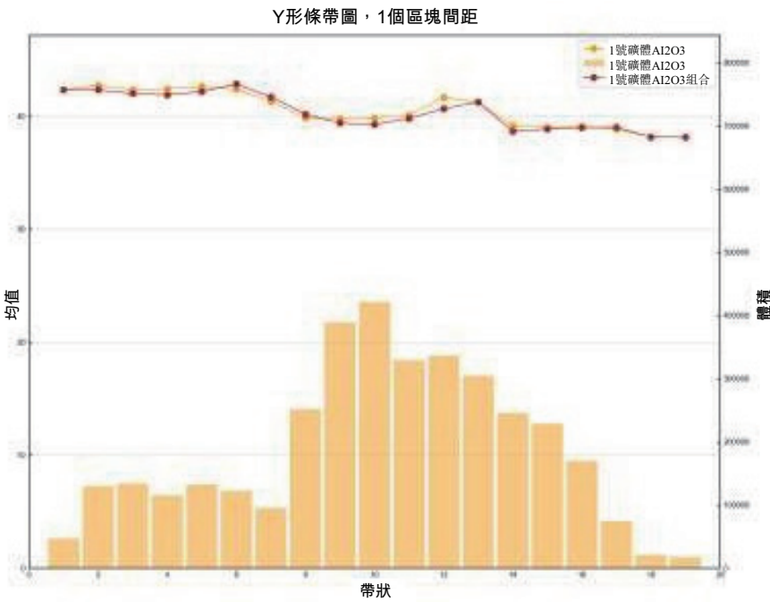
圖7.8：北至南向條帶圖－1號礦體
