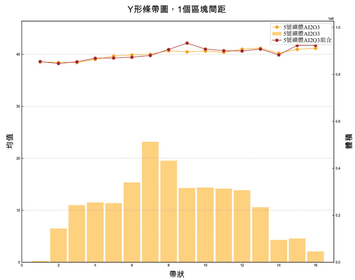
圖7.6：北至南向條帶圖－5號礦體
