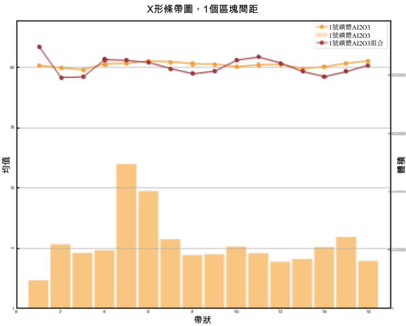
圖7.7：東至西向條帶圖－1號礦體
