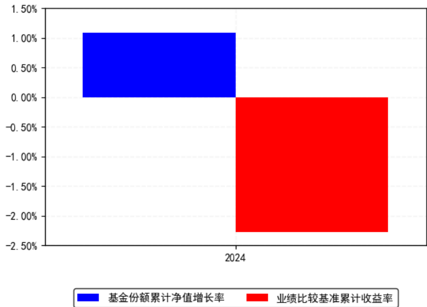
南方产业智选股票C每年净值增长率与同期业绩比较基准收益率的对比图（2024年12月31日）
