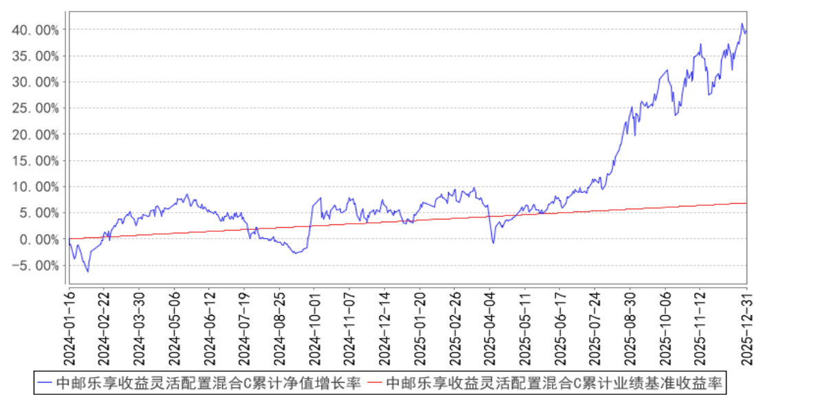
中邮乐享收益灵活配置混合C累计净值增长率与同期业绩比较基准收益率的历史走势对比图
