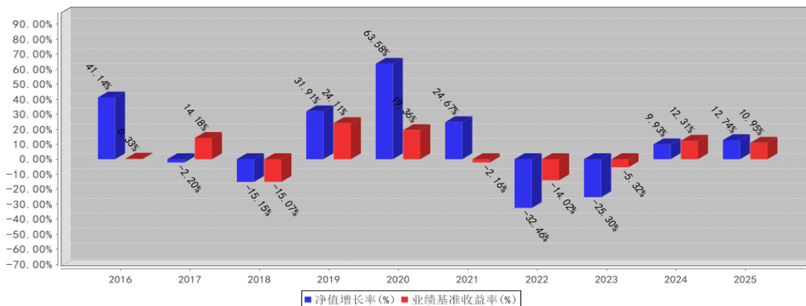
新沃通盈灵活配置混合基金每年净值增长率与同期业绩比较基准收益率的对比图 (2025年12月31日)
