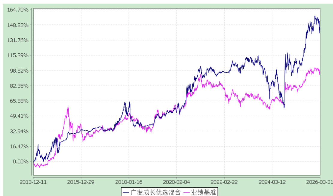
广发成长优选灵活配置混合型证券投资基金 累计净值增长率与业绩比较基准收益率历史走势对比图 (2013 年 12 月 11 日至 2026 年 3 月 31 日)
