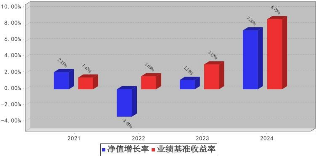
工银双玺6个月持有期债券C基金每年净值增长率与同期业绩比较基准收益率的对比图 (2024年12月31日)
