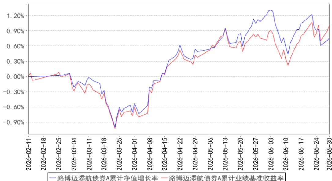
路博迈添航债券A累计净值增长率与同期业绩比较基准收益率的历史走势对比图
