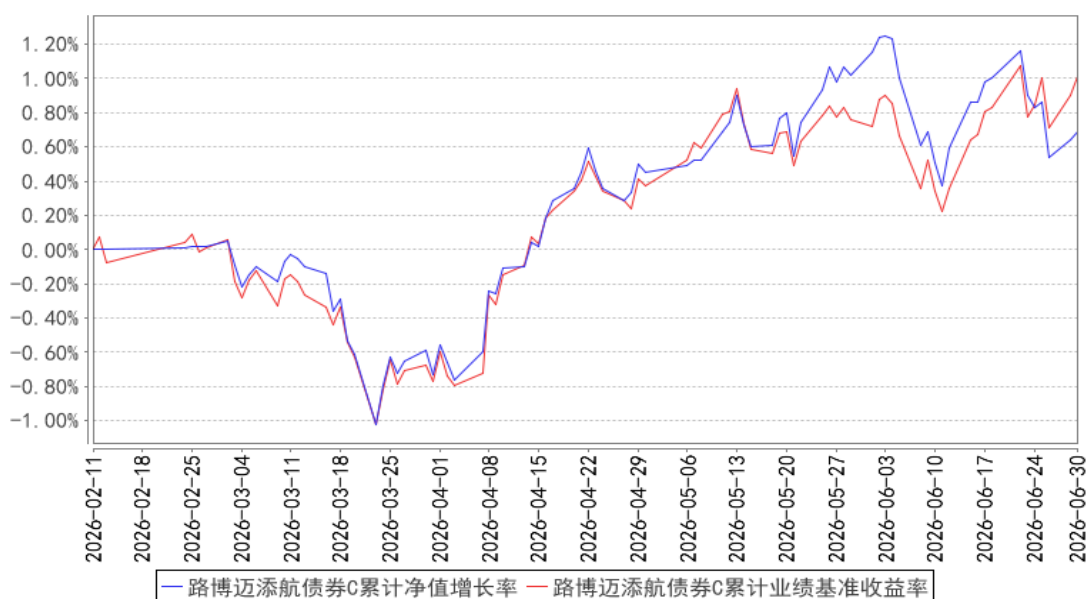
路博迈添航债券C累计净值增长率与同期业绩比较基准收益率的历史走势对比图
