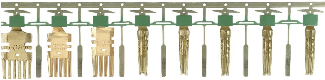
卷制接触件技术卷制过程示意图
