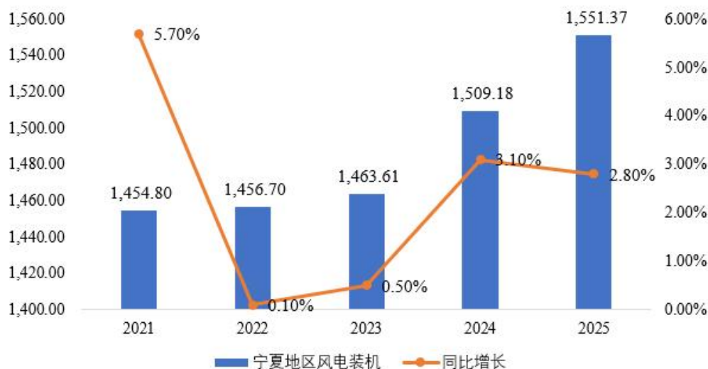
图表 3-16： 2021 年-2025 年宁夏地区风电装机情况
