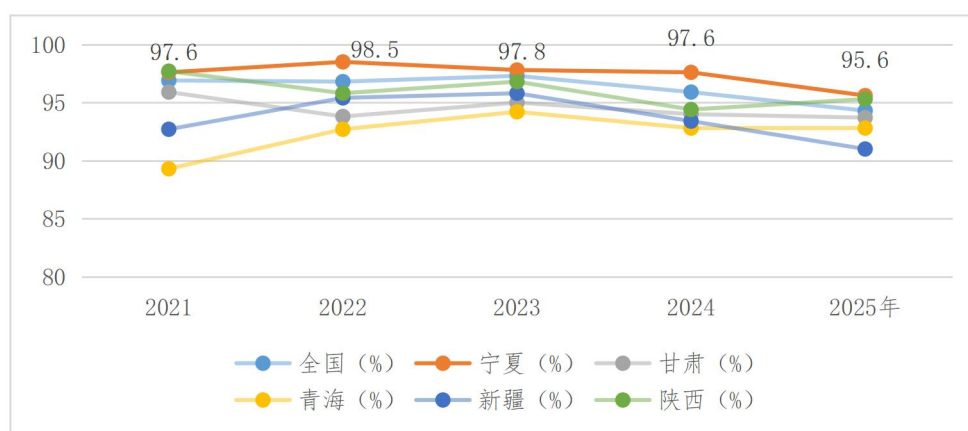
图表 3-122： 西北五省及全国 2021 年-2025 年风电利用率情况
