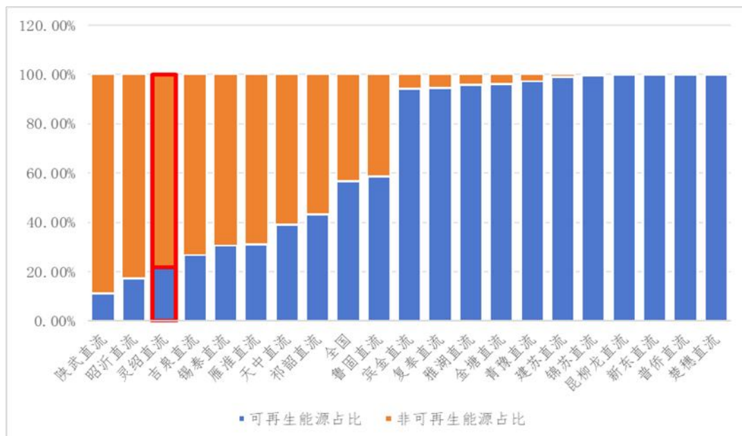
图表 3-16：2024 年直流特高压线路可再生能源占比
