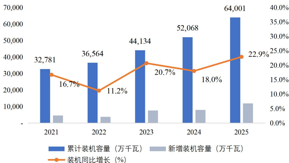
图表 2-20：2021-2025 年全国风电新增装机情况
