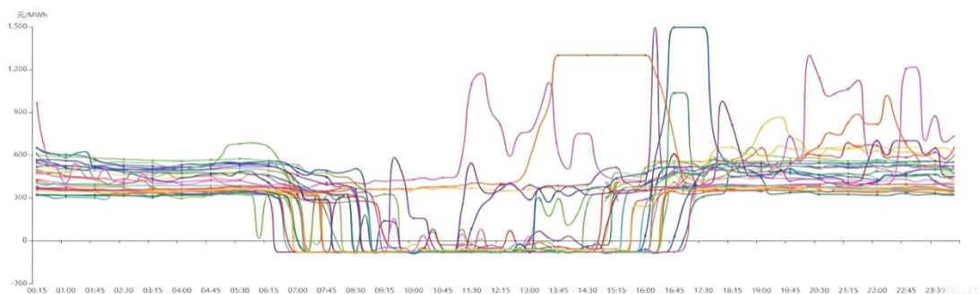
图表 3-38：2026 年 5 月 1 日-31 日山东省现货市场实时出清价格
