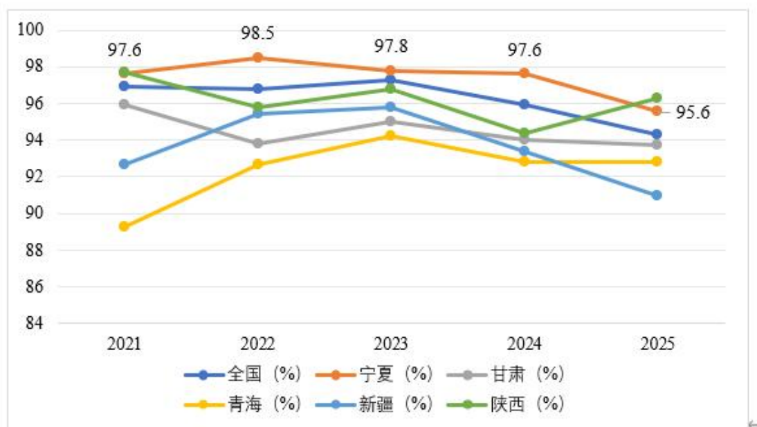
图表 3-17: 西北五省及全国 2021 年-2025 年风电利用率情况
