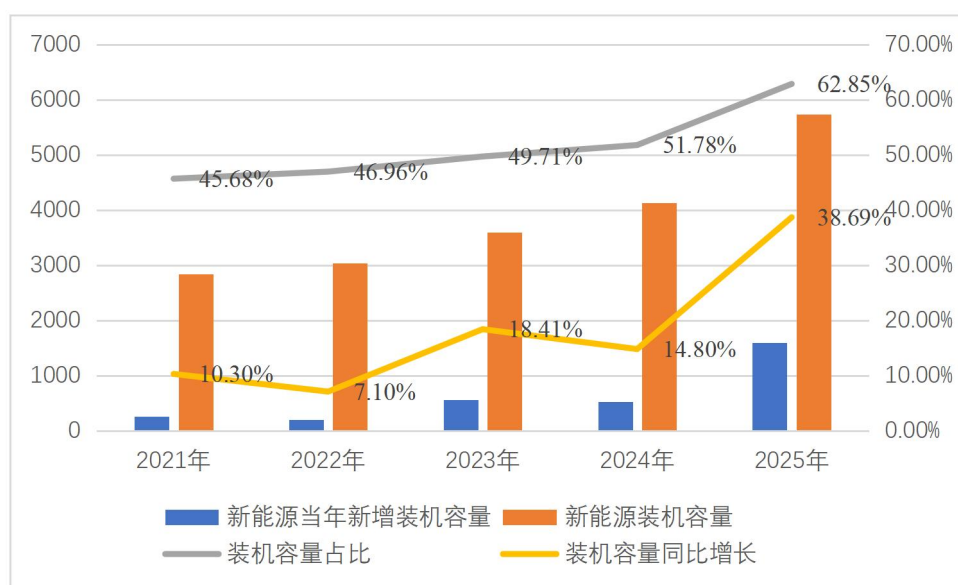
图表 3-36：宁夏新能源装机规模历史增长情况
