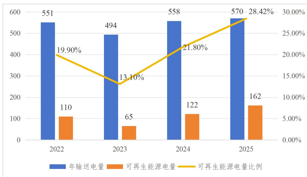
图表 2-16：2022 年-2025 年灵绍直流送出电量情况
