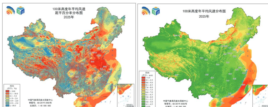
图表 3-15： 2025 年全国陆地 100 米高度年平均风速及风功率密度分布
