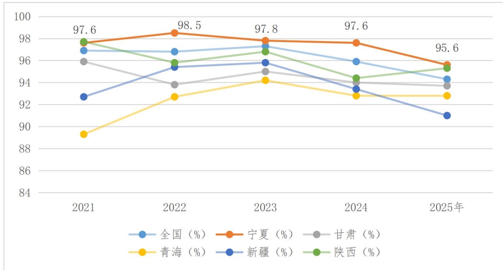
图表 3-44：西北五省及全国 2021 年-2025 年风电利用率情况
