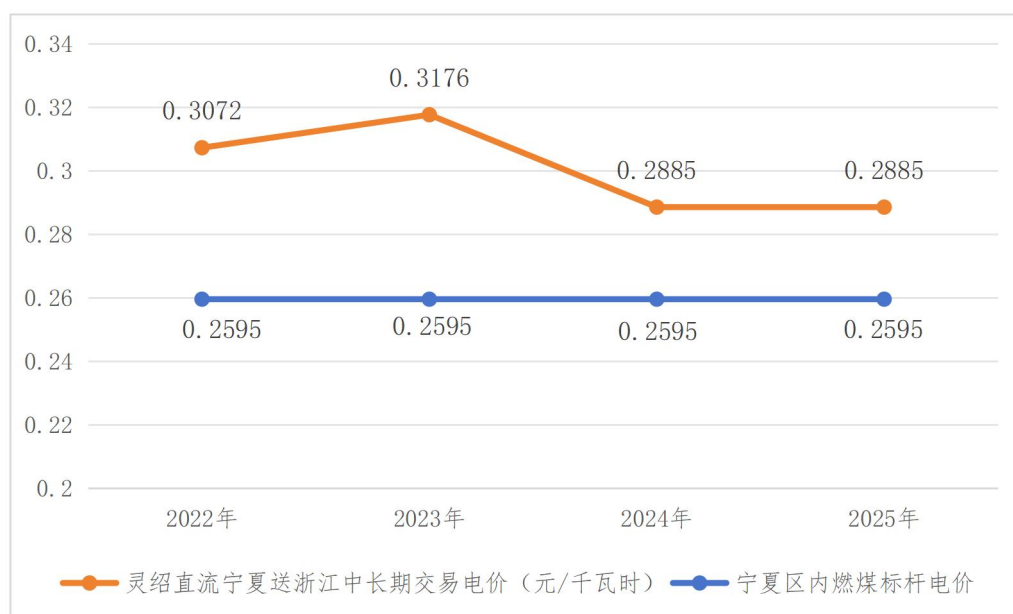
图表 3-24： 宁夏地区新能源通过灵绍直流送电浙江的中长期交易价格与宁夏区内燃煤标杆电价对比
