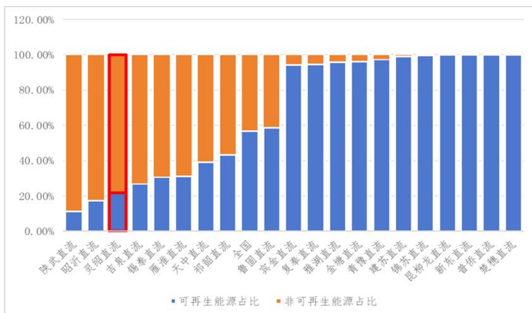
图表 3-94: 2024 年直流特高压线路可再生能源占比
