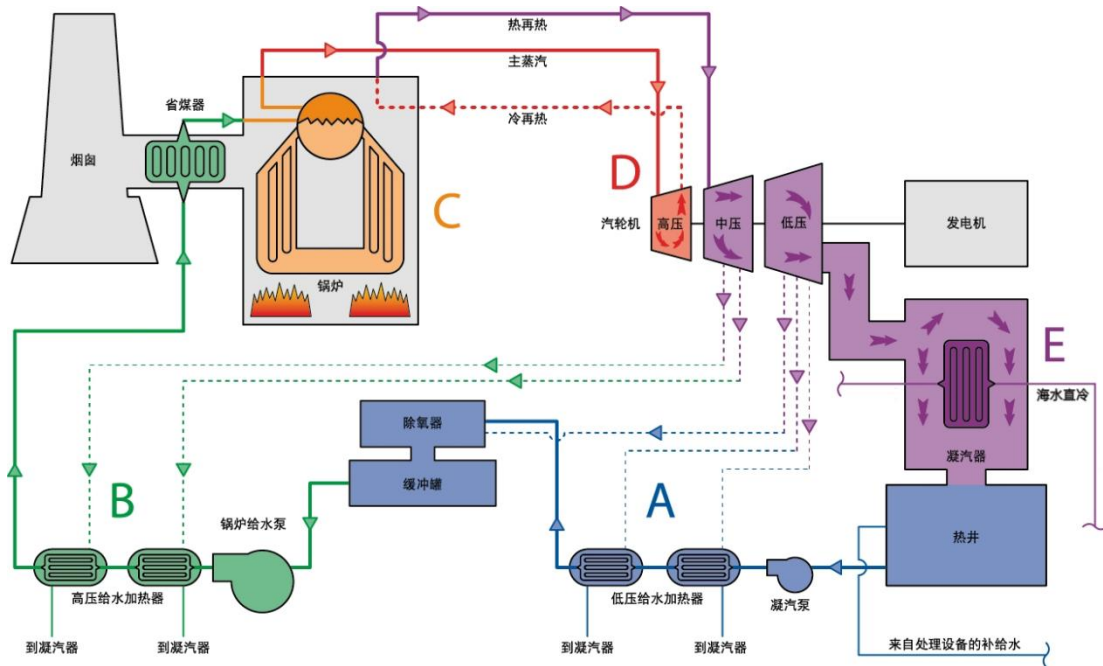
图表 2-19：燃煤热电联产机组生产工艺流程示意图
