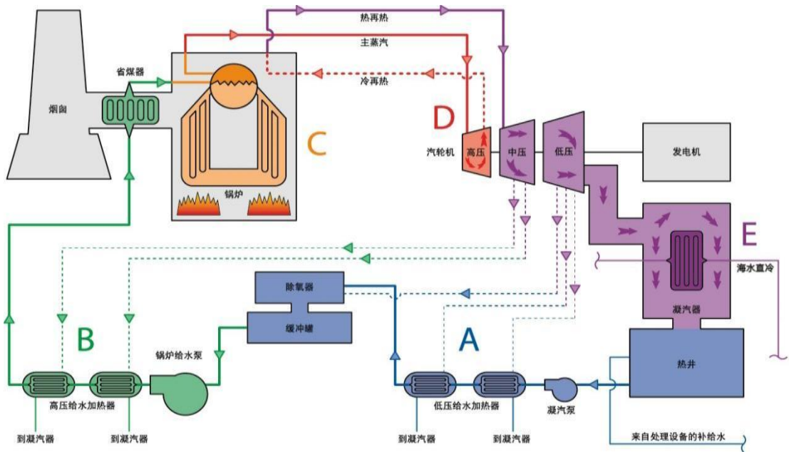
图表 3-3：燃煤热电联产机组生产工艺流程示意图
