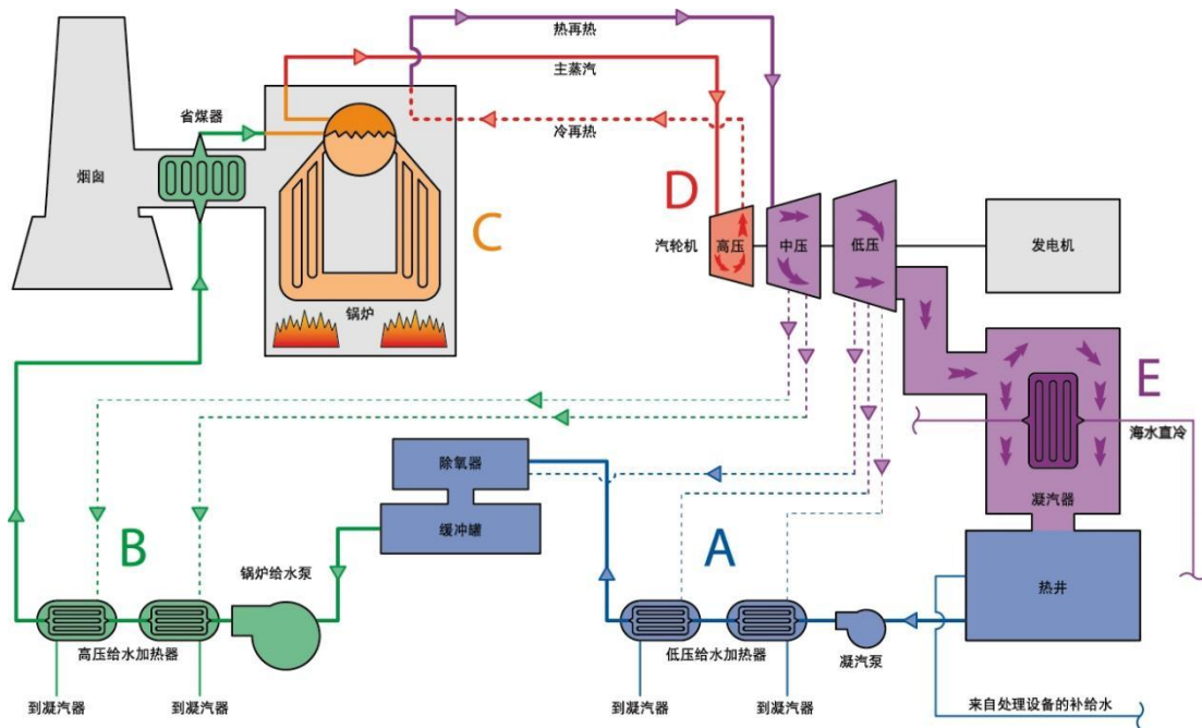
图：燃煤热电联产机组生产工艺流程图
