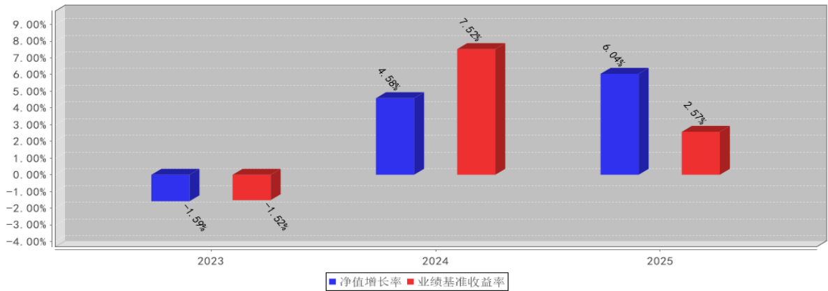
东方红共赢甄选一年持有混合C基金每年净值增长率与同期业绩比较基准收益率的对比图（2025年12月31日）
