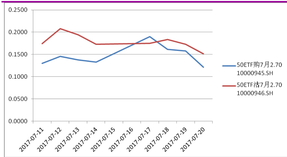
图表 10：7 月平值认购期权与平值认沽期权隐含波动率变化图（标准合约） （50ETF 购 7 月 2700）VS（50ETF 沽 7 月 2700）
