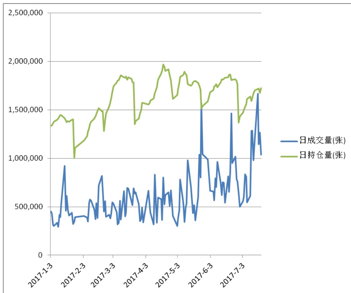
图表 6：上证 50ETF 期权自 2017 年以来日成交量和日持仓量变化图
