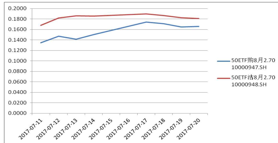
图表 14：8 月平值认购期权与平值认沽期权隐含波动率变化图（标准合约） （50ETF 购 8 月 2700）VS（50ETF 沽 8 月 2700）
