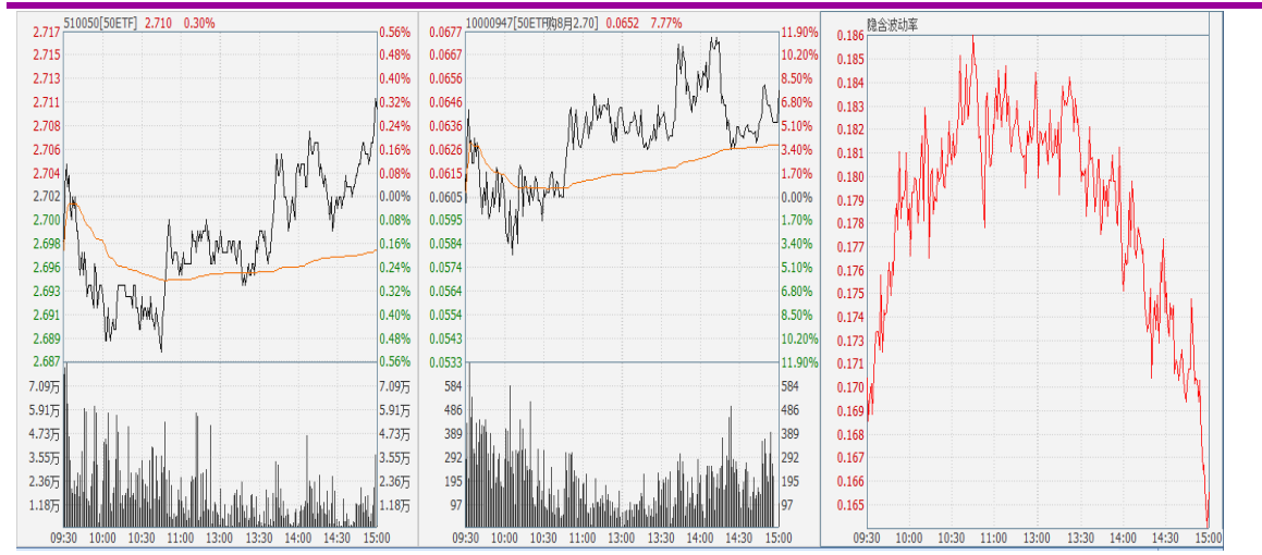
图表 12：50ETF 与 8 月平值认购期权“50ETF 购 8 月 2700”日内走势图及隐含波动率走势图
