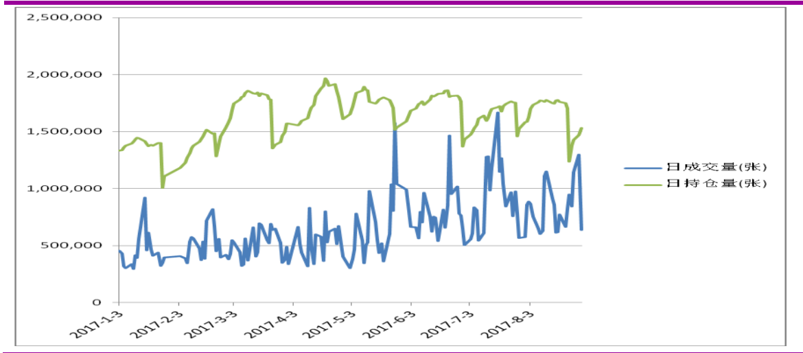
图表 6：上证 50ETF 期权自 2017 年以来日成交量和日持仓量变化图
