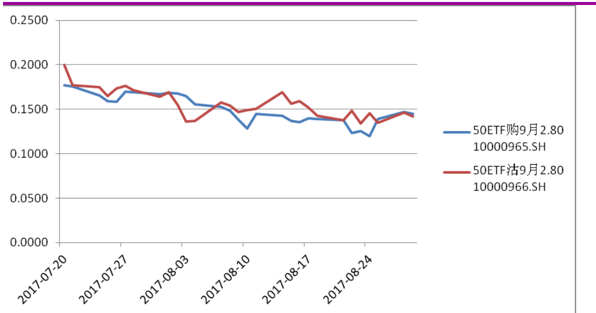
图表 10：9 月平值认购期权与平值认沽期权隐含波动率变化图 ( 50ETF 购 9 月 2800 ) VS ( 50ETF 沽 9 月 2800 )
