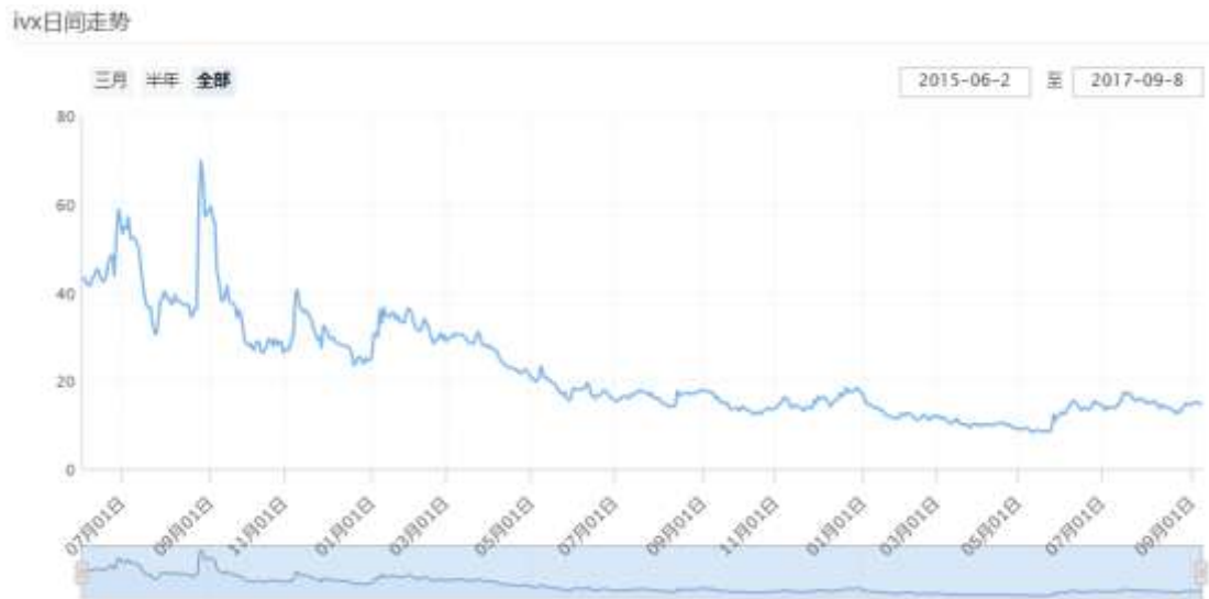
图表 13：中国波指的日间走势（全部）
