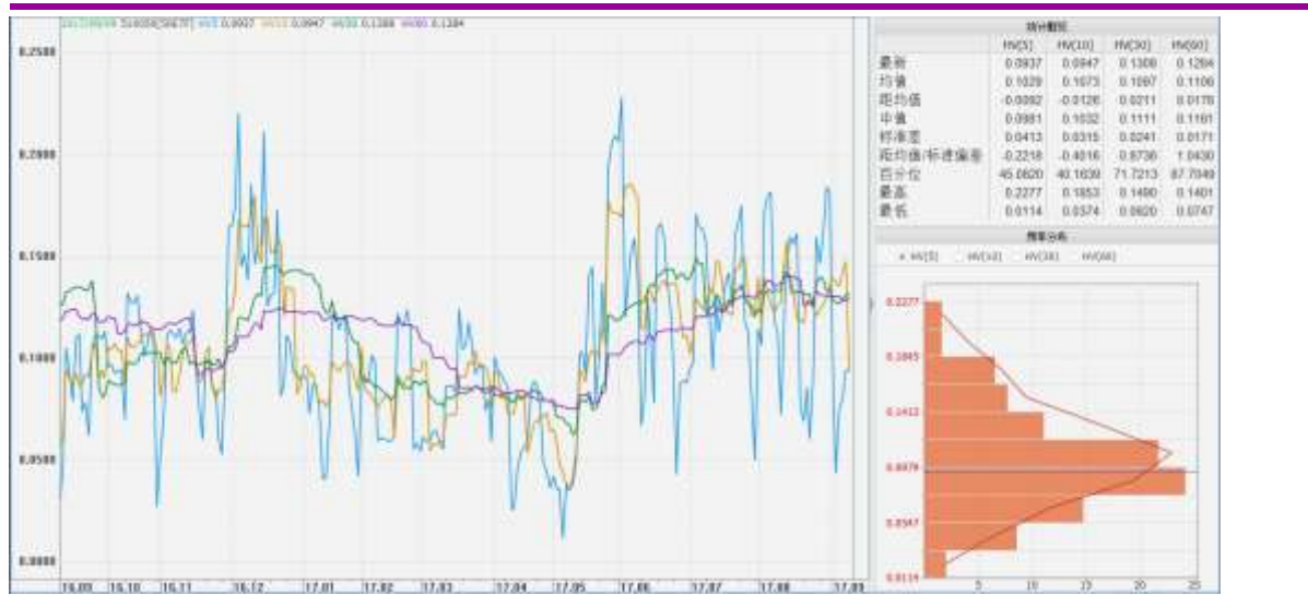
图表 15：上证 50ETF 最近 1 年的历史波动率变化图（参数为 5 日、10 日、30 日、60 日）
