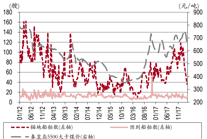
图表 8. 秦皇岛港锚地船舶与煤价走势
