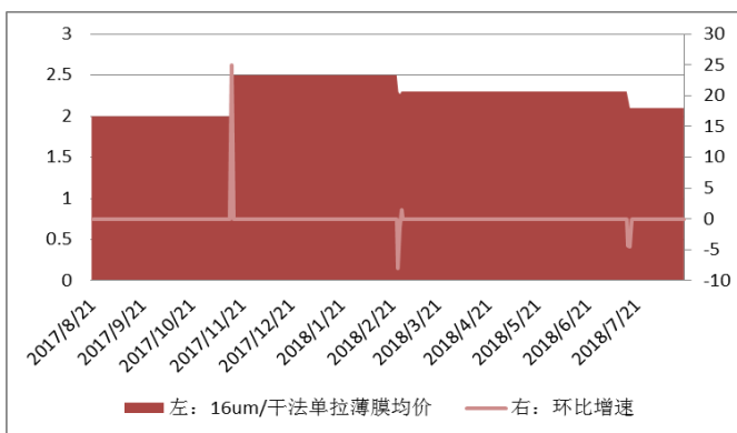
图 17: 干法单拉薄膜国内价格走势 (元/平方米, %)
