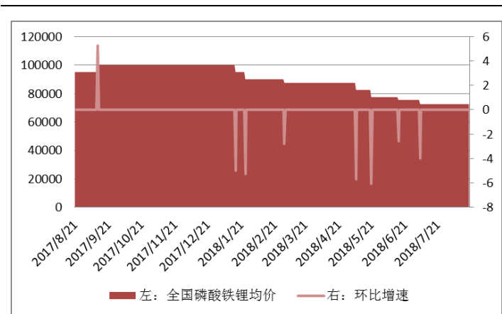
图 11：磷酸铁锂国内价格走势（元/吨，%）
