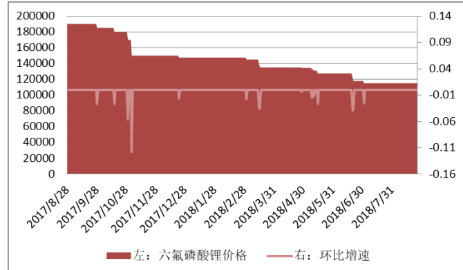
图 14：六氟磷酸铁锂价格走势（元/吨，%）
