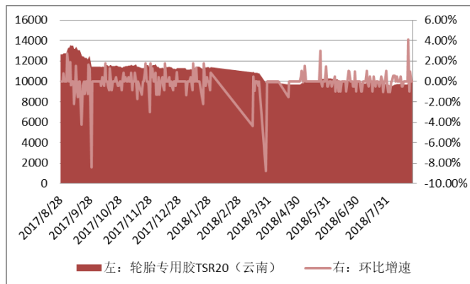
图 9：轮胎专用胶市场价格走势（元/吨，%）
