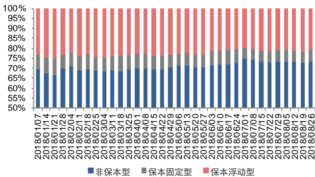
图 2：新发行理财产品中非保本型占比上升
