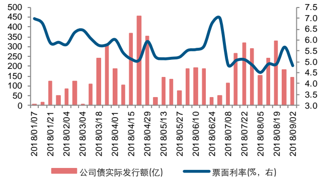
图 8：公司债发行规模继续下降，利率回落
