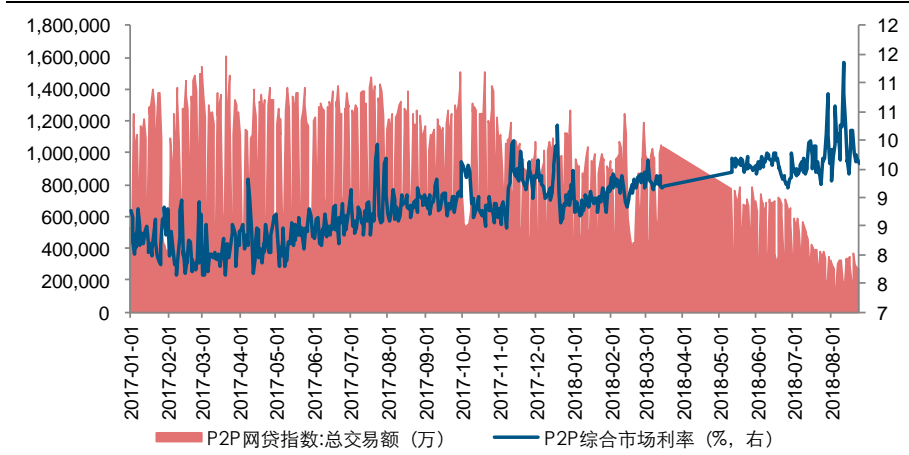
图 11: P2P 成交额略有增加, 利率下降
