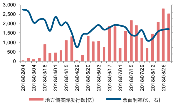
图 7：地方债发行有所回落，但维持高位，利率继续上行
