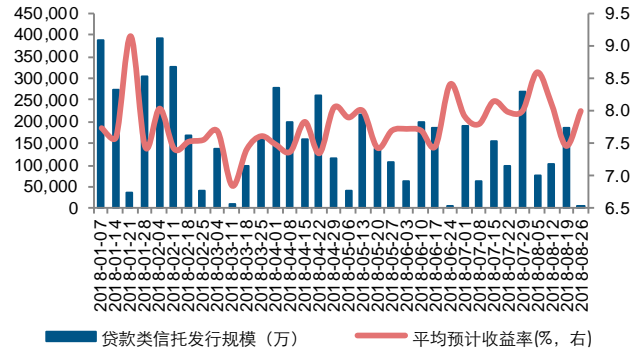
图 5：新成立贷款类信托规模略增加，利率继续下降
