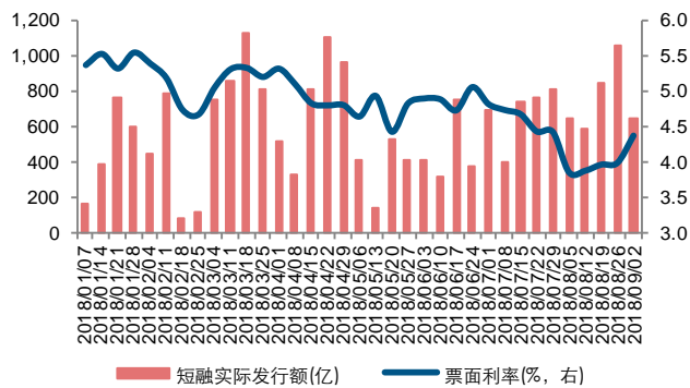
图 9：短融发行规模显著减少，利率继续上升
