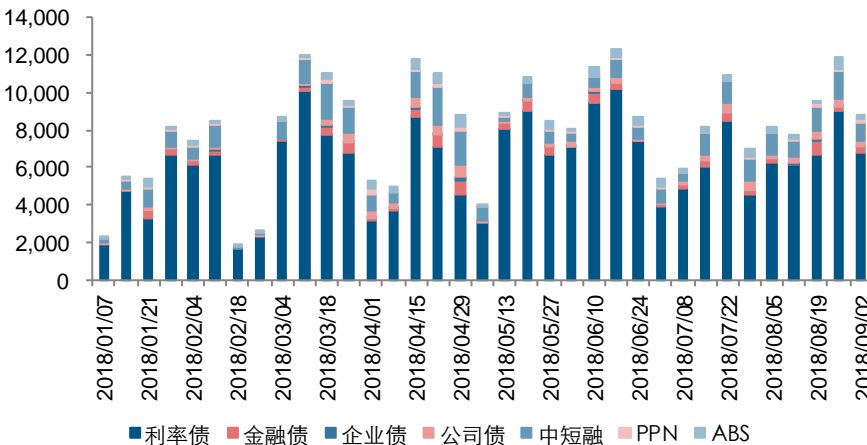
图 6：债券发行量回落（单位：亿）
