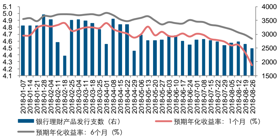
图 1：银行新发行理财产品数量减少，预期年化收益率下降
