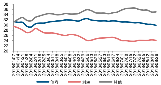
图 3：理财产品债券配置比例有所下降（单位：%）
