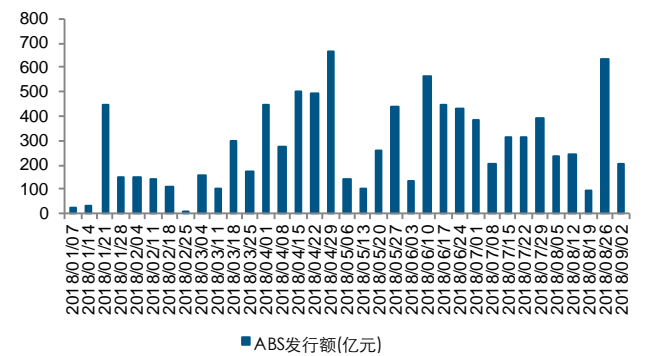
图 10：ABS 发行规模显著回落
