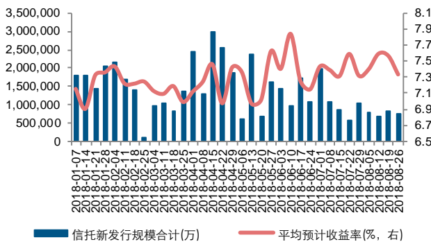
图 4：信托新发行规模续降，但降幅趋缓，利率继续回升
