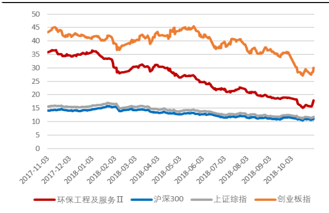
图 5: PE (TTM)
