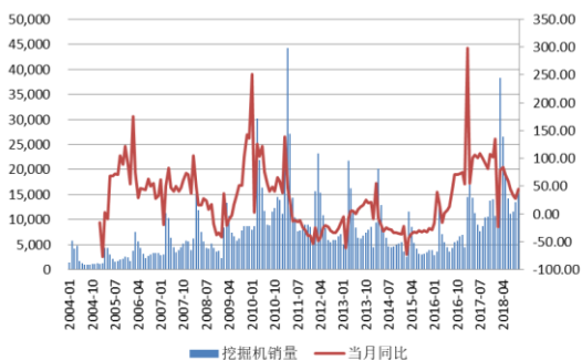
图 1：主要企业挖掘机销量及同比变动（台，%）
