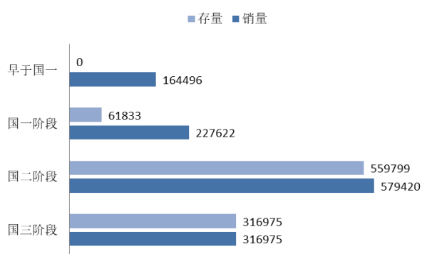
图 8：不同排放阶段挖掘机销量及存量（台）
