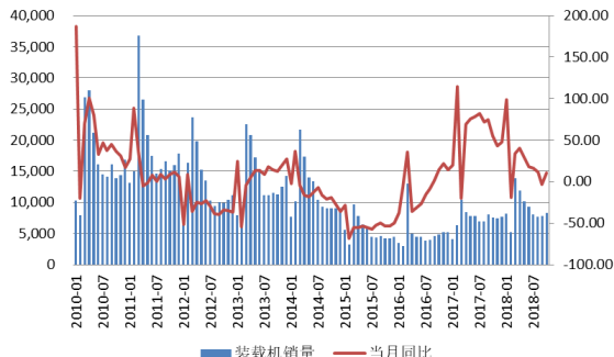
图 2：主要企业装载机销量及同比变动（台，%）
