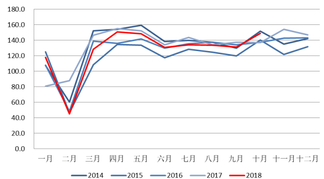
图 7：小松挖掘机中国地区开机小时数
