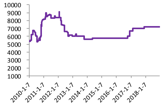
图表44: 冰晶石价格走势 (元/吨)
