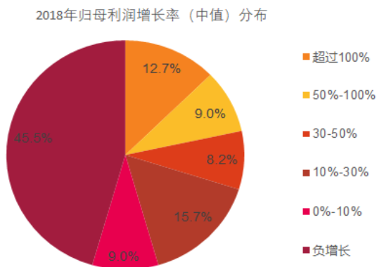
图 5：2018 年 134 家公司归母净利润增长率（中值）分布
