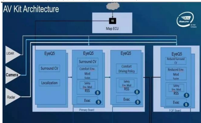
图表18 英特尔自动驾驶完整硬件系统
