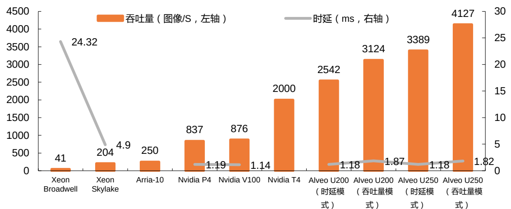
图表10 赛灵思 FPGA 产品图像吞吐量和时延指标表现优异
