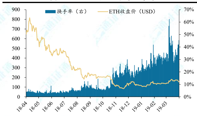
图表10: ETH 收盘价与换手率
