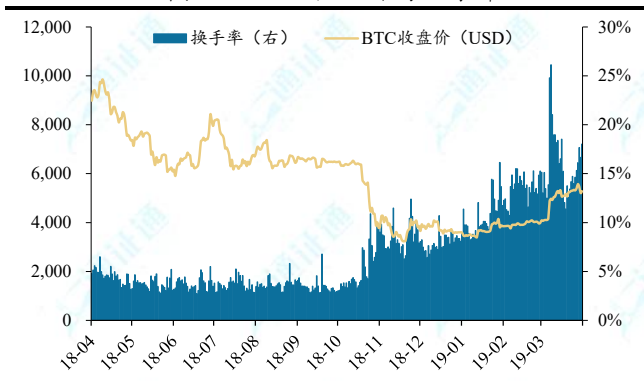
图表9: BTC 收盘价与换手率
