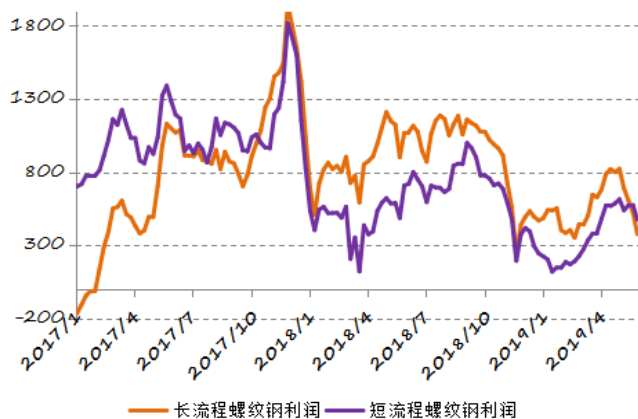
图 5：长短流程螺纹钢利润走势（元/吨）
