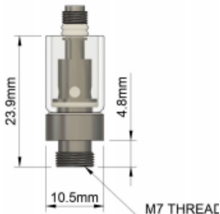
图：用于CBD雾化器的cCELL雾化芯孔径为10.5mm
