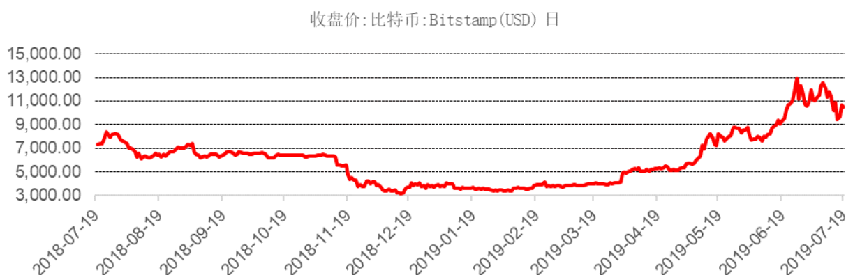
图表11： 比特币价格
