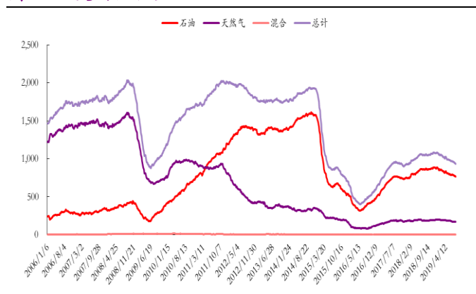
图 33: 美国钻机数
