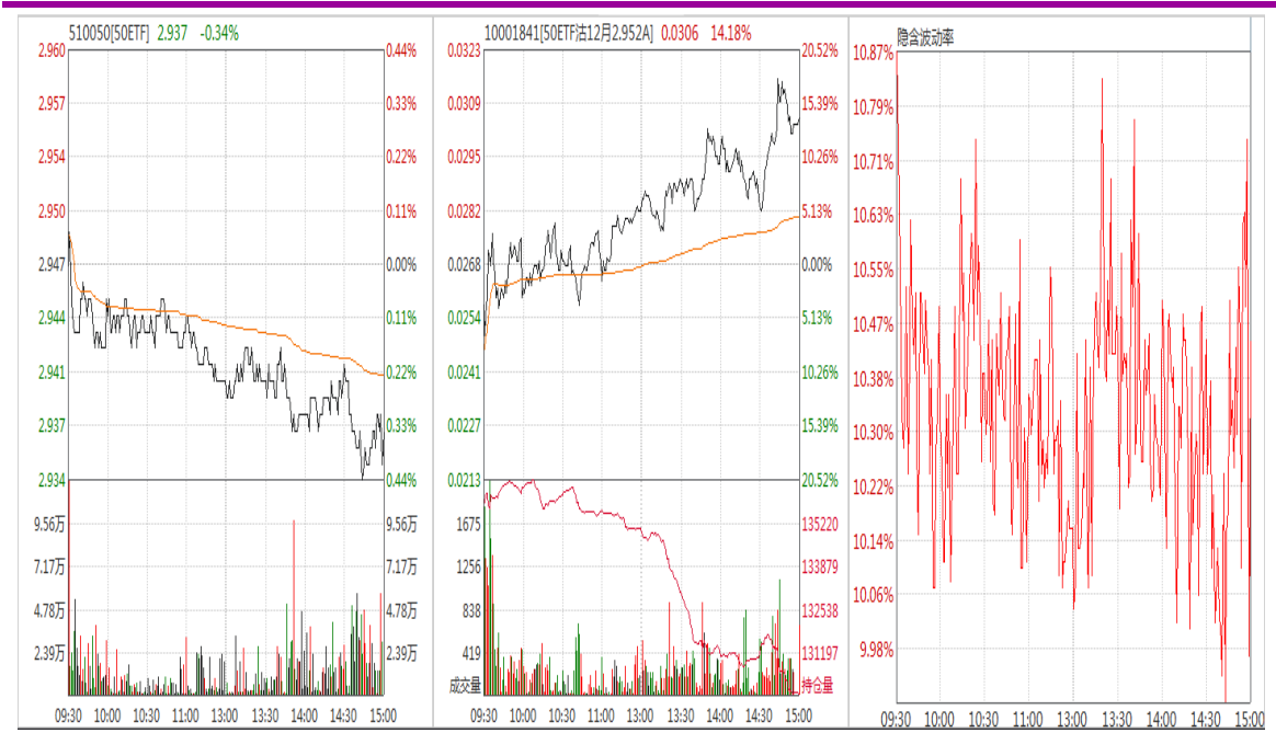
图表 10：50ETF 与 12 月平值认沽期权“50ETF 沽 12 月 2952A”日内走势图及隐含波动率走势图
