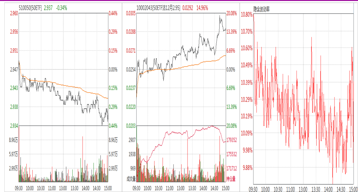
图7：50ETF与12月平值认沽期权“50ETF沽12月2950”日内走势图及隐含波动率走势图
