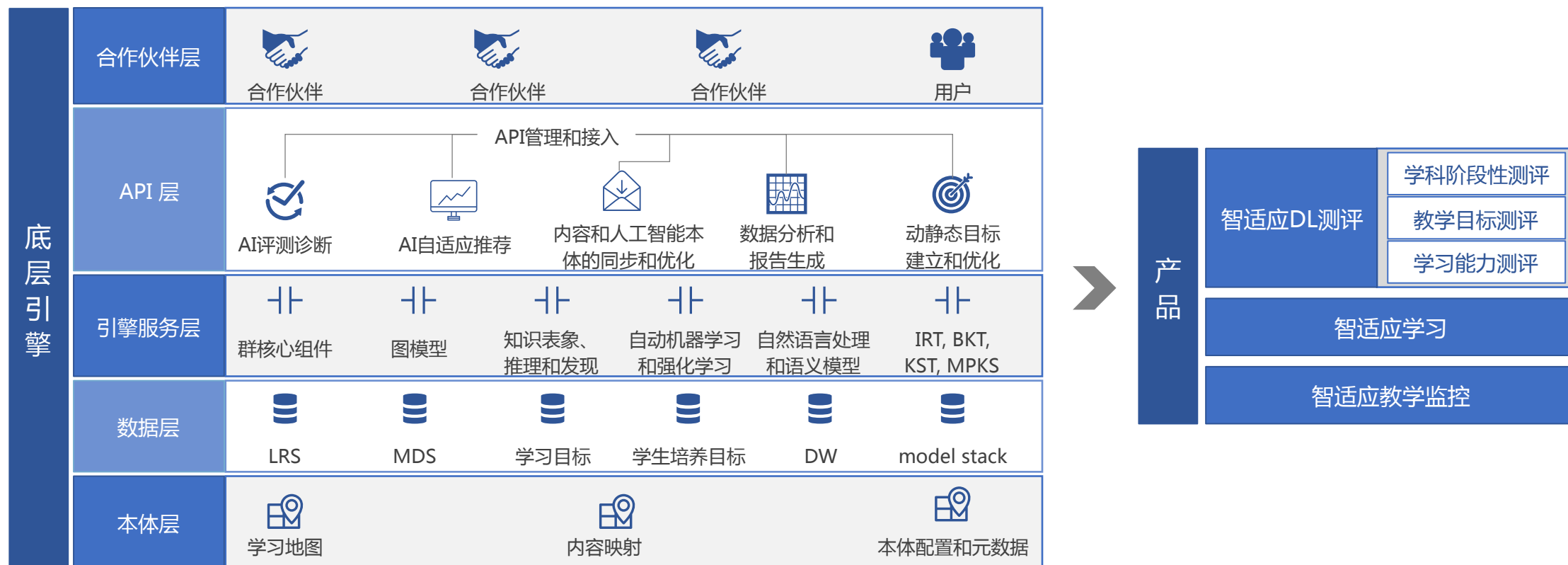
松鼠AI智适应教育开放平台的底层引擎
