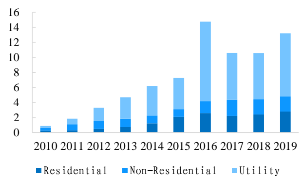
图3: 户用是美国光伏装机的重要构成
