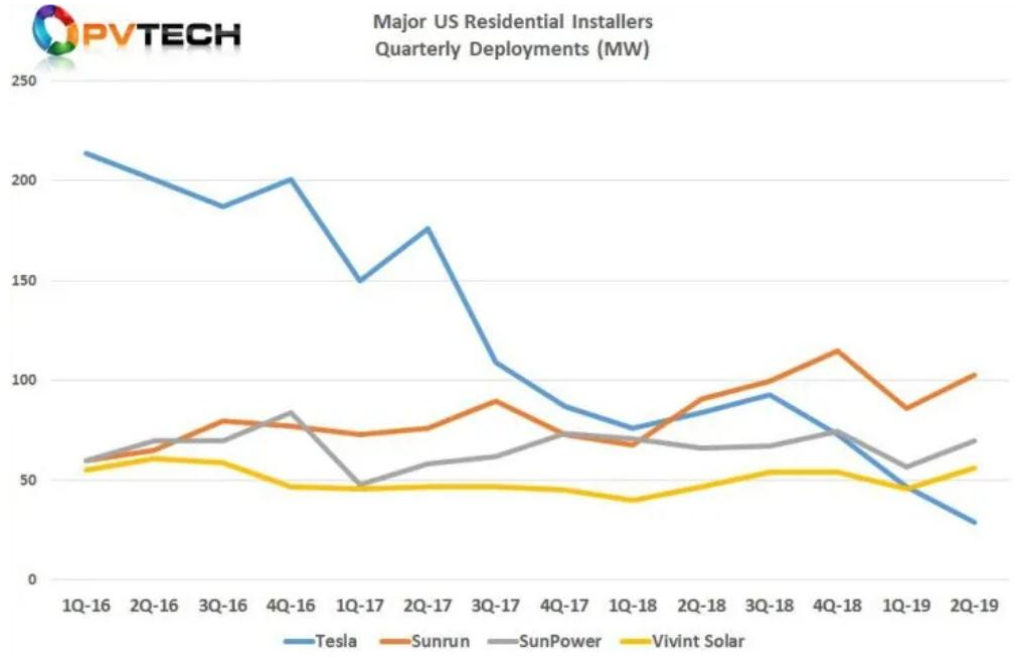
图1: Sunrun 与 Vivint Solar 分别是美国排名第一、第三的户用光伏安装商
