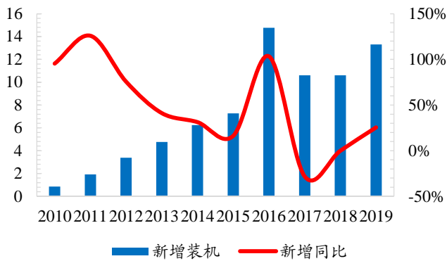
图2: 美国光伏装机稳定增长
